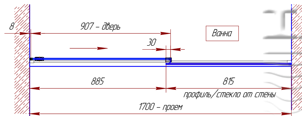
Перегородка в закрытом состоянии
