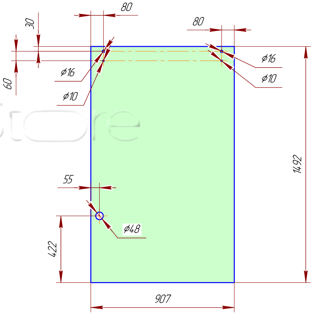
Дверь поз.2, 1 штука
