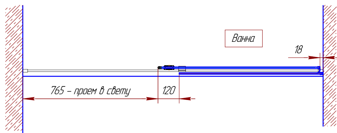
Перегородка в открытом состоянии
